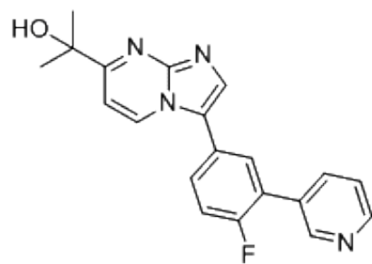
PC-6277001, DMSO-d 6
